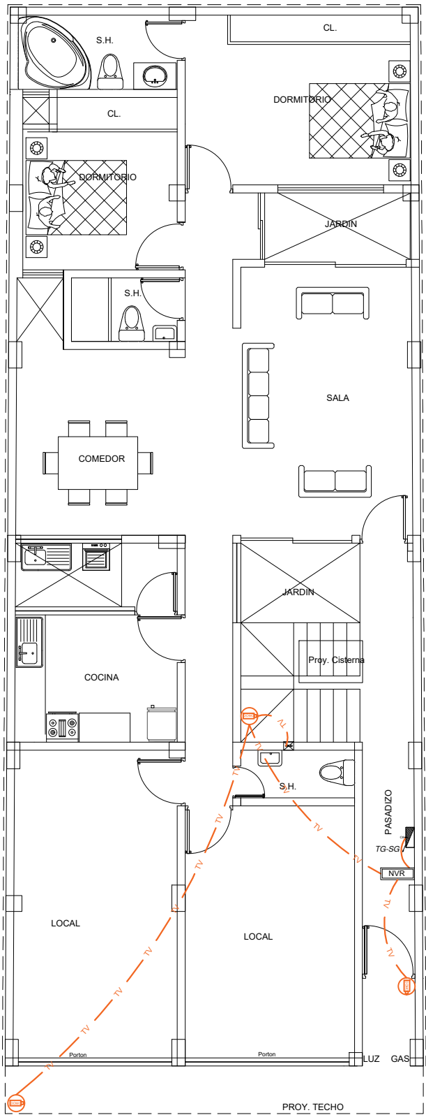
PRIMERA PLANTA
